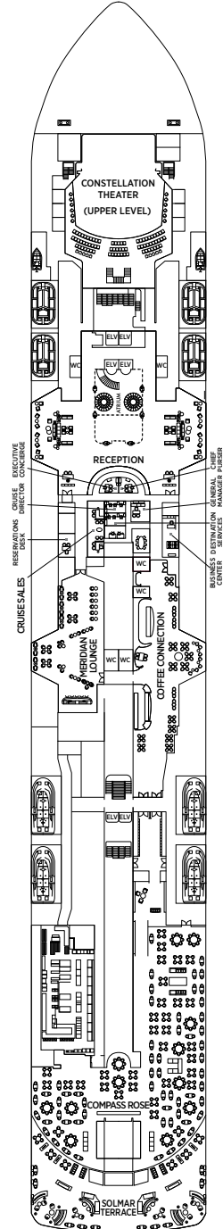
CUBIERTA 5
