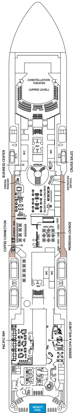
CUBIERTA 5
